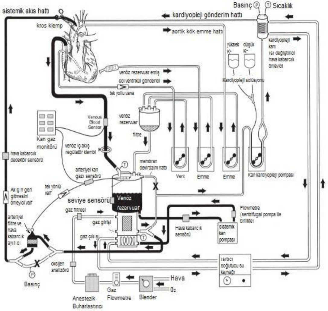
Şekil 1. Vücut dışı (ekstrakorporeal dolaşım) devresi (24).
