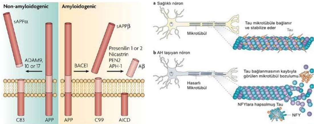
Şekil 4.2: APP'nin \alpha , \beta ve \gamma sekretazlarla amiloidojenik ve amiloidojenik olmayan proteoliz işlemi (A); sağlıklı nöronlarda ve taupati durumunda tau proteini (B)
