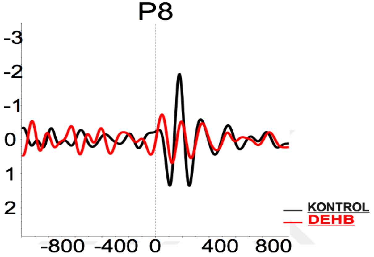
Şekil 6.7. İki grubun P8 elektrodundan kızgın yüz ifadesi uyarısına verdiği teta (4-7 Hz) osilatuar yanıtının büyük ortalamaları
