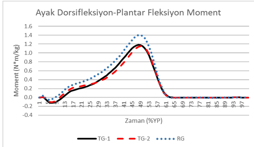
Şekil 6-5: Alt ekstremitte sagittal plan moment grafikleri. TG-1: Tabanlık Grubu tabanlıksız yürüyüş verileri, TG-2: Tabanlık Grubu tabanlıklılı yürüyüş verileri RG: Referans grubu yürüyüş verileri, %YP: yürüyüş periyodu yüzdesi
