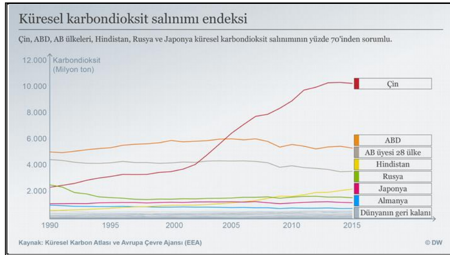
Grafik 23. 2015 Yılı Küresel Karbondioksit Salınım Endeksi
