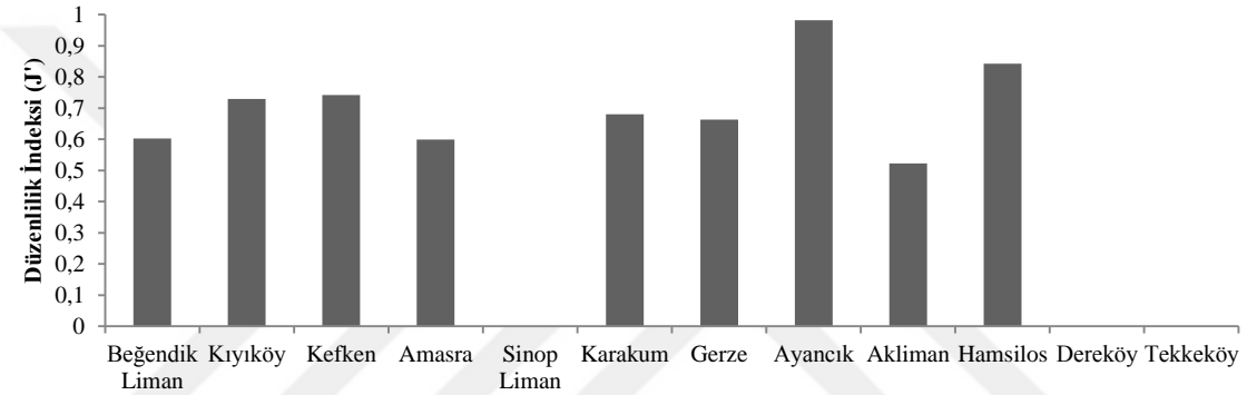
Şekil 20. İstasyonlara göre düzenlilik indeksi değerleri.
