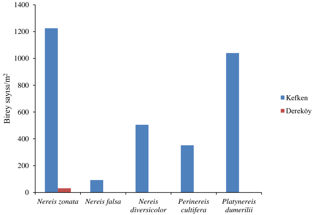
Şekil 23. Mytilus galloprovincialis fasiesinde türlerin dağılımı.
