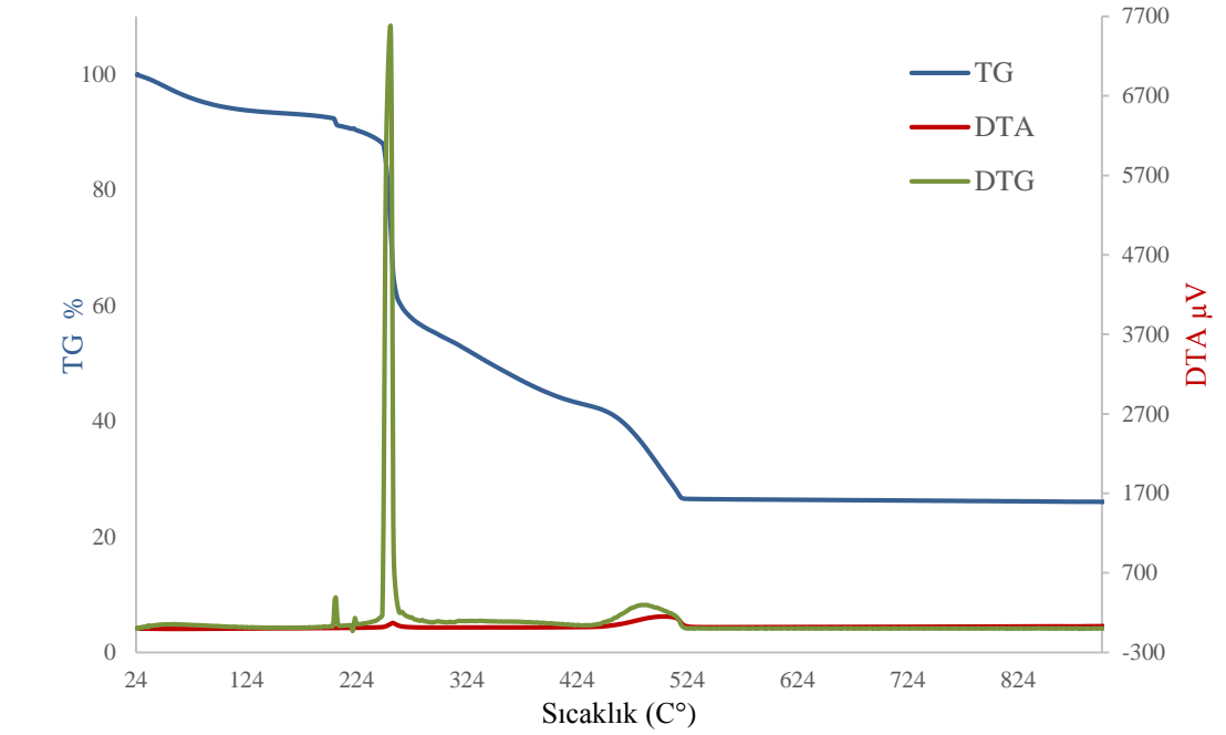
Şekil 87. [Cu(FIAH)(OH)]·H 2 O kompleksine ait termik analiz eğrileri
