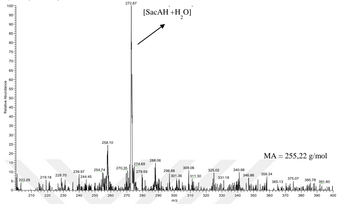
Şekil 83. SacAH-Na molekülüne ait kütle spektrumu
