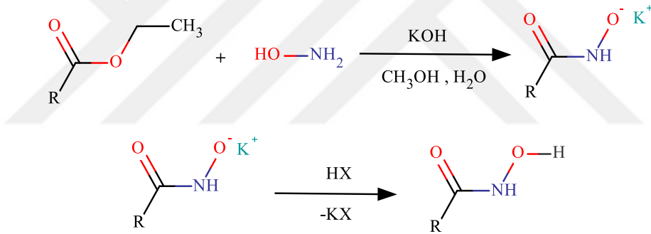
Şekil 2. Blatt yöntemiyle hidroksamik asit sentezi
