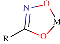
Şekil 21. Enol formundaki hidroksamik asidin metal kompleksinin yapısı
