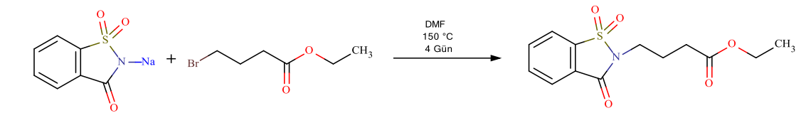
Şekil 38. Etil sakkarin-N-bütanoat Sentezi
