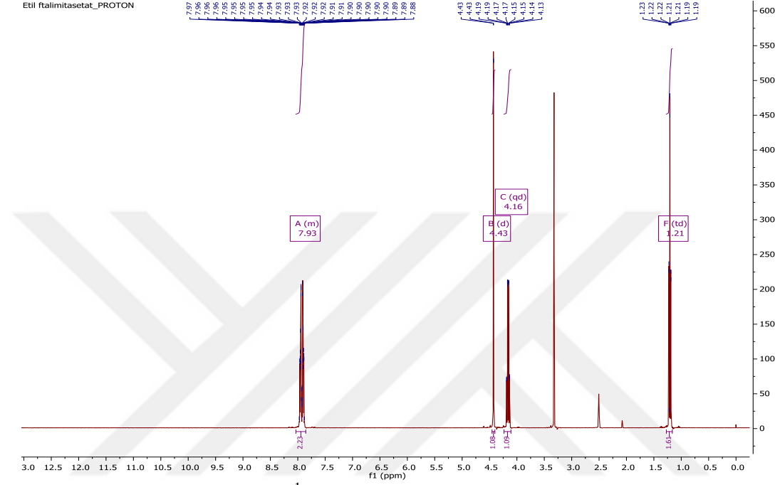
Şekil 67. EFIA molekülüne ait ^1\text{H} -NMR spektrumu
