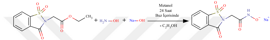
Şekil 37. Sodyum sakkarin-N-asetohidroksamat tuzu sentezi
