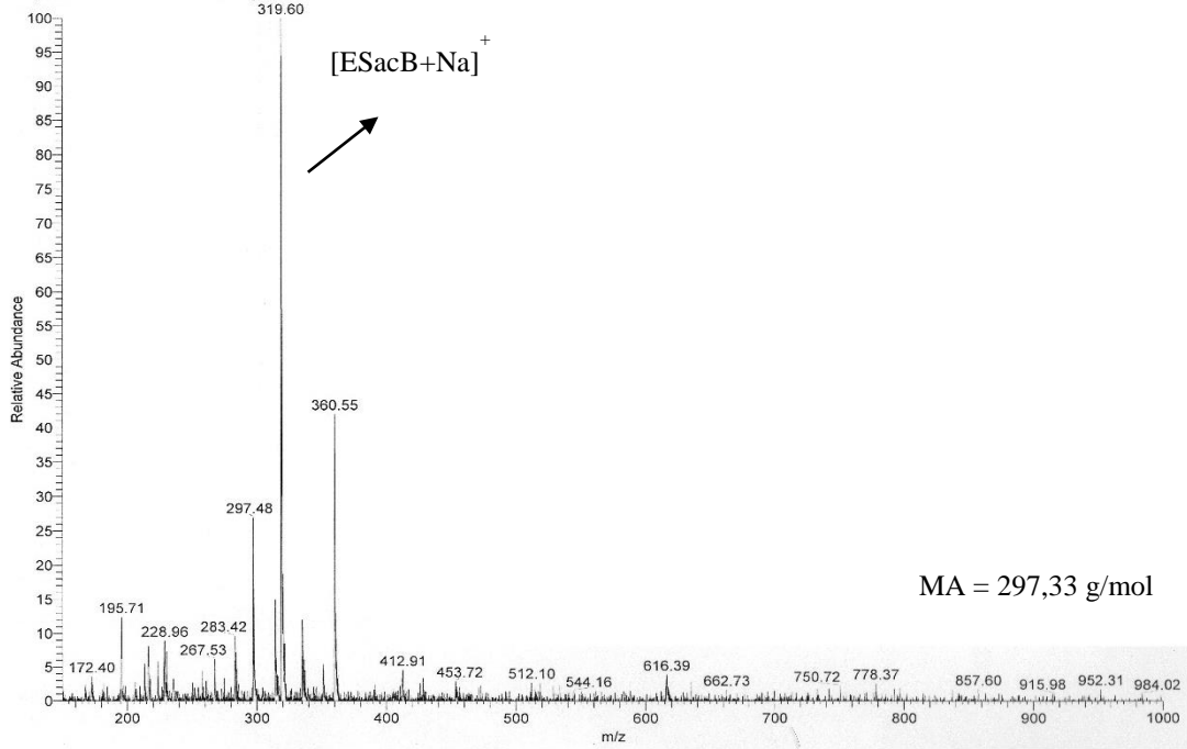
Şekil 84. ESacB molekülüne ait kütle spektrumu
