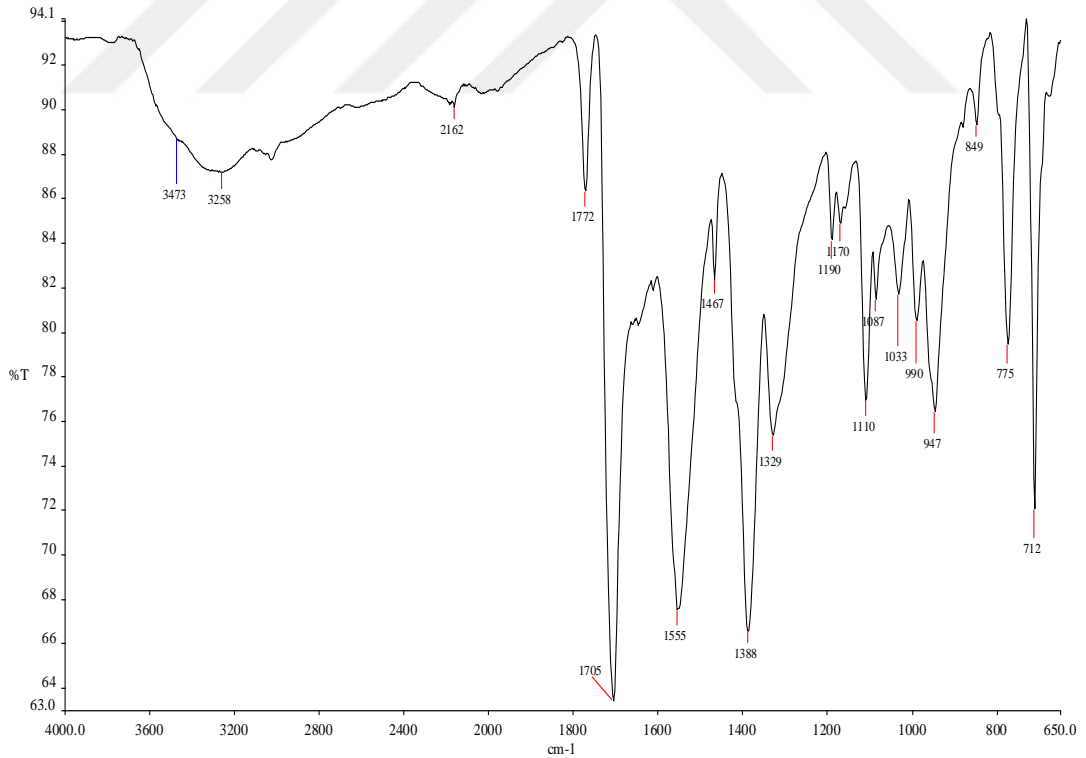
Şekil 45. [\text{Cu}(\text{FIAH})(\text{OH})] \cdot \text{H}_2\text{O} kompleksine ait IR spektrumu
