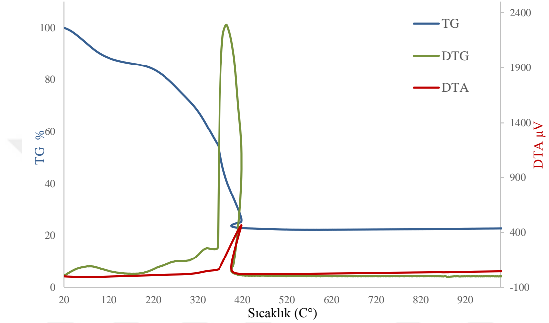
Şekil 86. [Ni(FIAH)(OH)]·2,5H 2 O kompleksine ait termik analiz eğrileri
