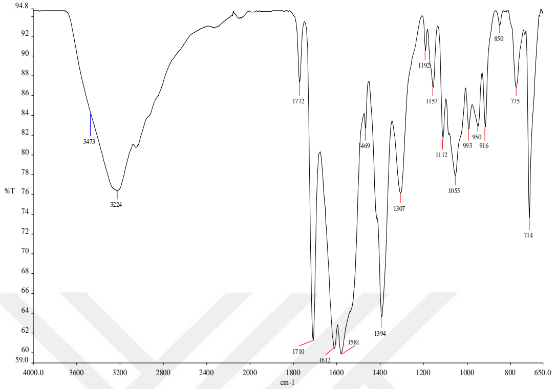
Şekil 44. [\text{Ni}(\text{FIAH})(\text{OH})] \cdot 2,5\text{H}_2\text{O} kompleksine ait IR spektrumu
