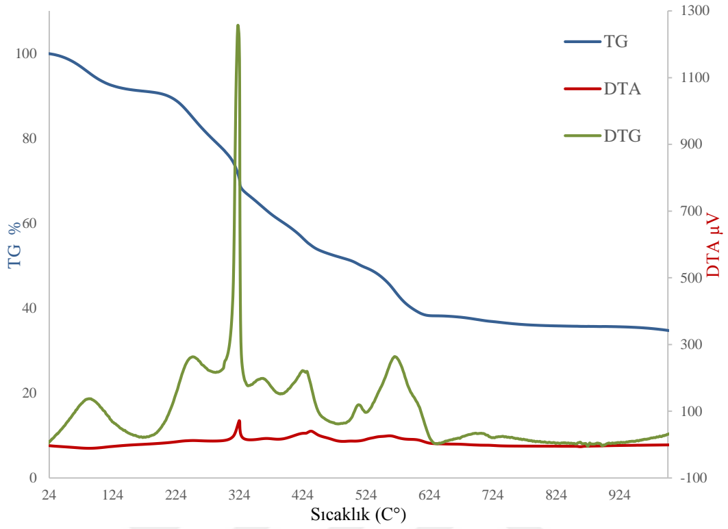
Şekil 94. [Cd(SacAH)(OH)] \cdot 2H_2O molekülüne ait termik analiz eğrileri
