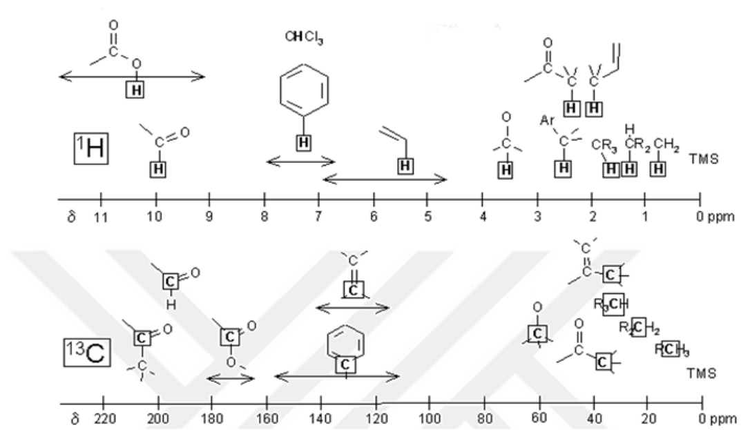
Şekil 33. Bazı grupların ^1\text{H} ve ^{13}\text{C} NMR kimyasal kayma aralıkları
