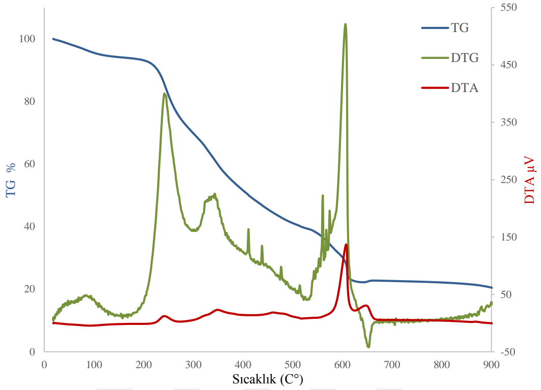
Şekil 98. [Zn(SacBH)(OH)] \cdot H_2O molekülüne ait termik analiz eğrileri
