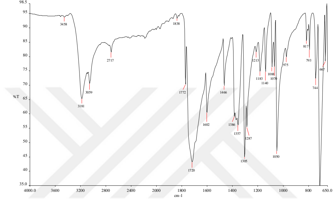
Şekil 40. Ftalimit molekülüne ait IR spektrumu
