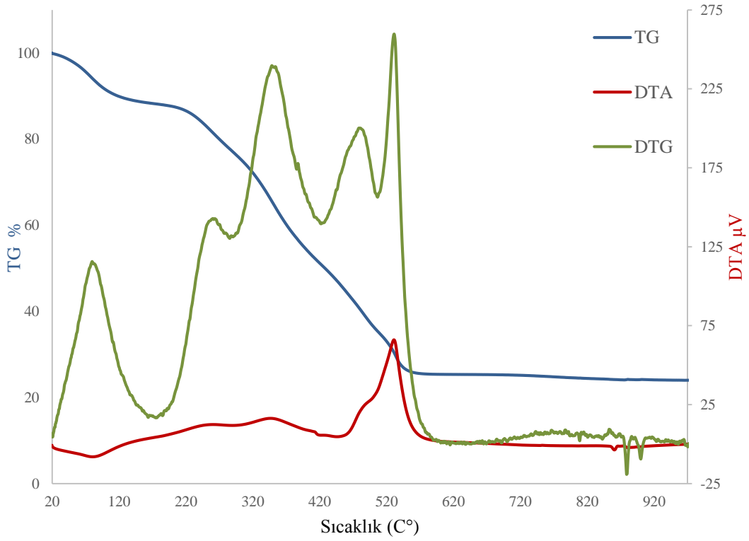
Şekil 93. [\text{Zn}(\text{SacAH})(\text{OH})]\cdot 2,5\text{H}_2\text{O} molekülüne ait termik analiz eğrileri
