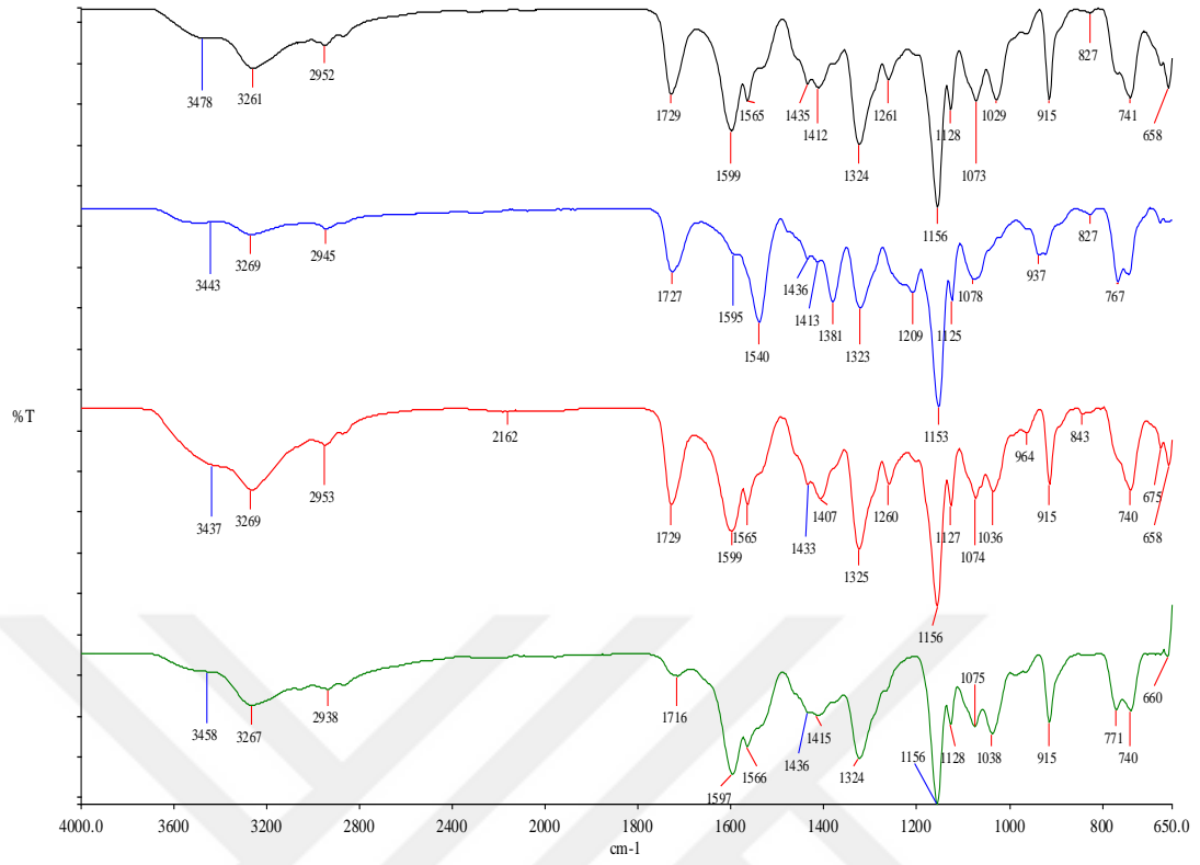
Şekil 66. SacBH–M komplekslerine ait IR spektrum karşılaştırılması
