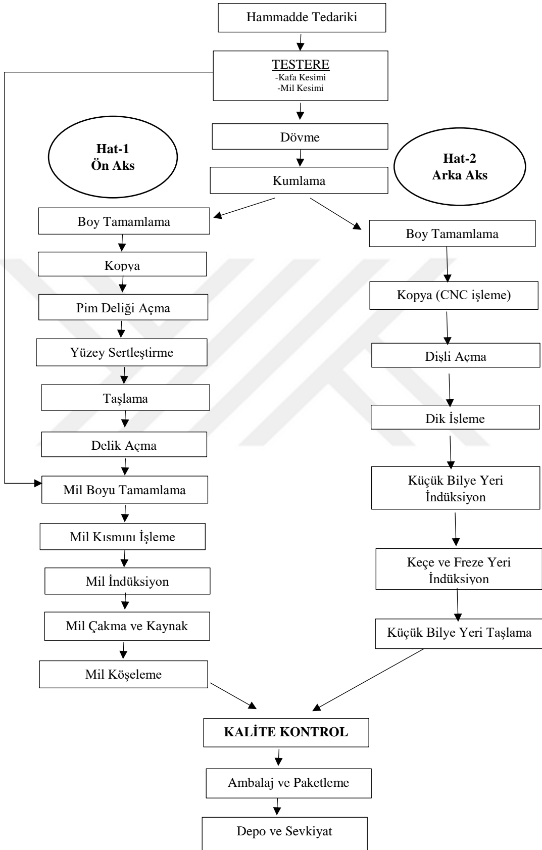
Şekil 14. MF Grubu Traktörlerin İş Akış Şeması
