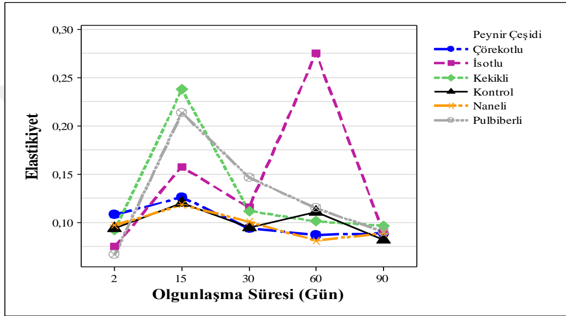
Şekil 4.4.7. Peynir örneklerinde elastikiyet yönünden peynir çeşidi x olgunlaşma süresi interaksiyonu
