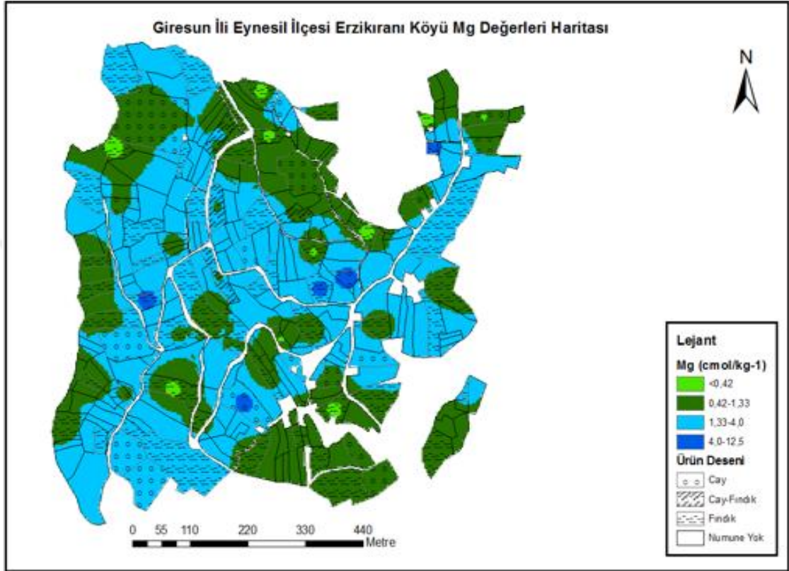
Şekil 4.10. Erzikıranı Köyü Mg değerleri IDW haritası
