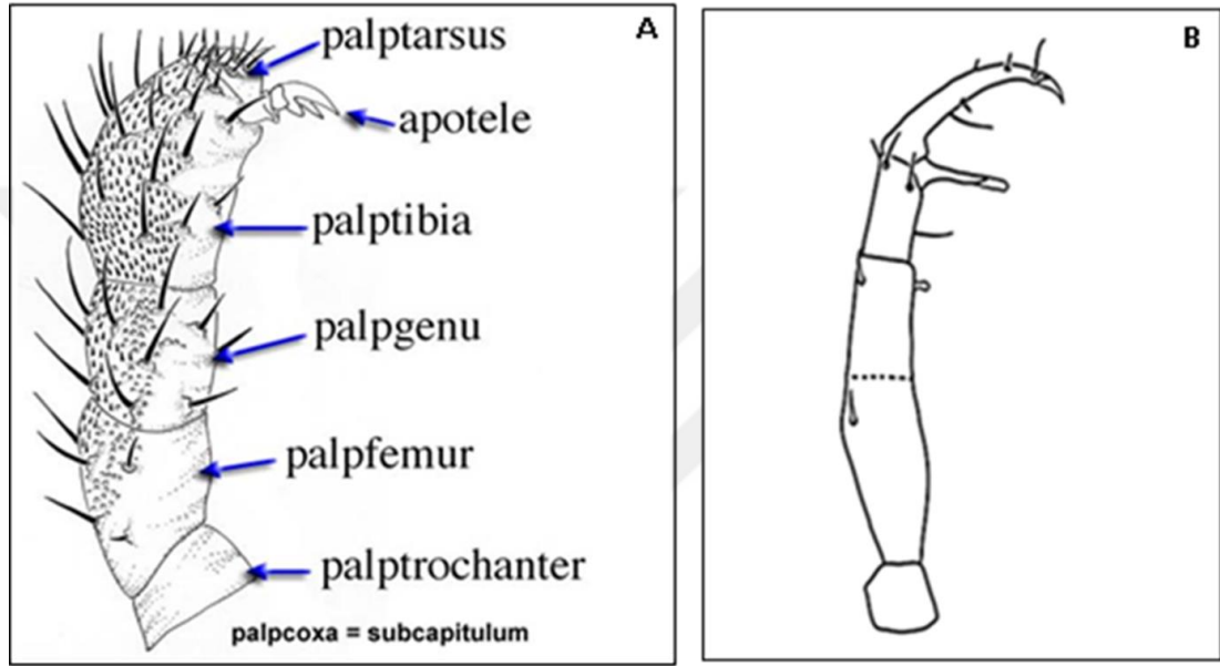
Şekil 3.5. Palpus segmentleri- Allothyryrus sp. (Holothyrida: Allothyridae) (A) (Walter, 2005) ve tutucu (raptorial) palp- Dactyloscirus sp. (Prostigmata: Cunaxidae) (B) (Skvarla ve ark., 2014)
