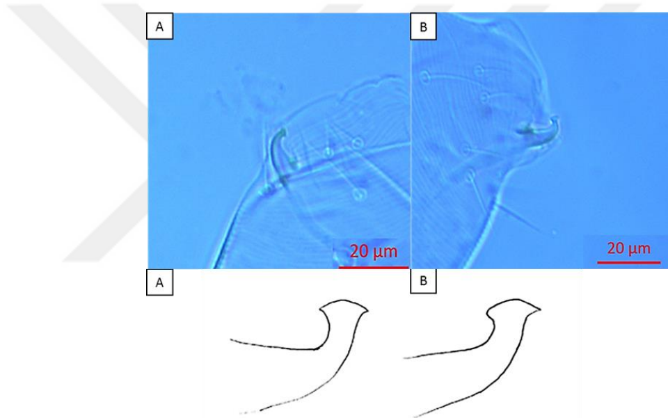
Şekil 4.7. Tetranychus urticae de aedeagus yapıları ( T. urticae , (A), T. urticae (kırmızı form) (B)) (Zhang, 2003)
