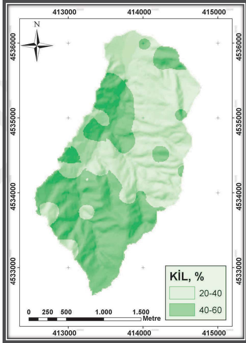
Şekil 4.6. Çalışma alanına ait % kil dağılım haritası
