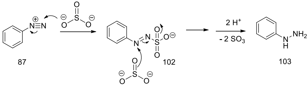
Şekil 1.48. Arilhidrazine (103) indirgenme
