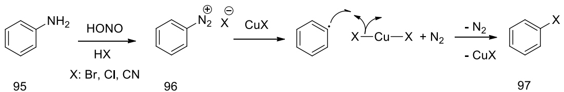
Şekil 1.45. Sandmayer reaksiyonu
