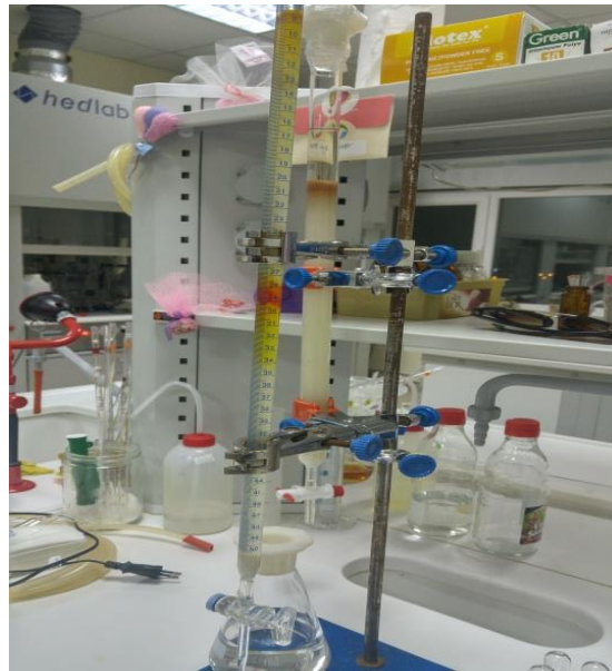
Şekil 4.60. Bileşik 6'nın kolon kromatografisi
