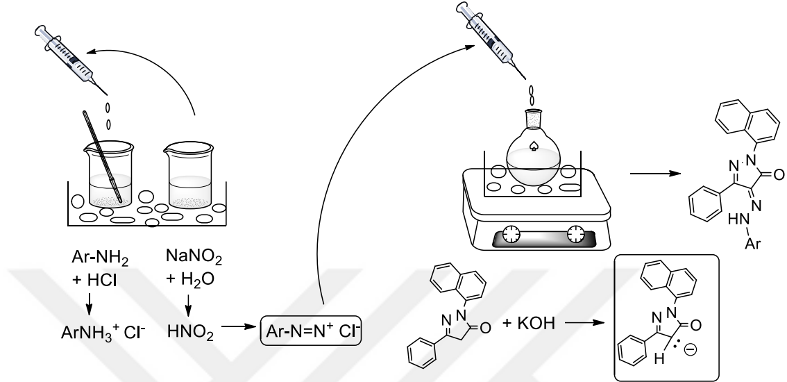
Şekil 5.3. Azo-5-pirazolonların hazırlanması
