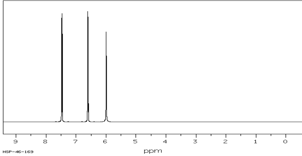
Şekil 4.18. 4,4'-Diaminodifenil sülfon bileşiğinin 1 H NMR spektrumu
