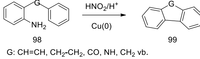
Şekil 1.46. Pschorr reaksiyonu
