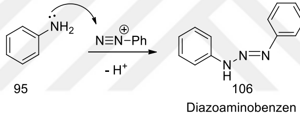
Şekil 1.50. Diazoaminobenzen (106) sentezi
