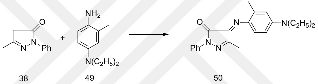
Şekil 1.22. Aminlerle reaksiyon
