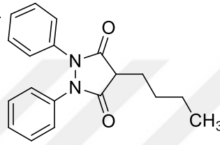
Fenilbütazon 74
