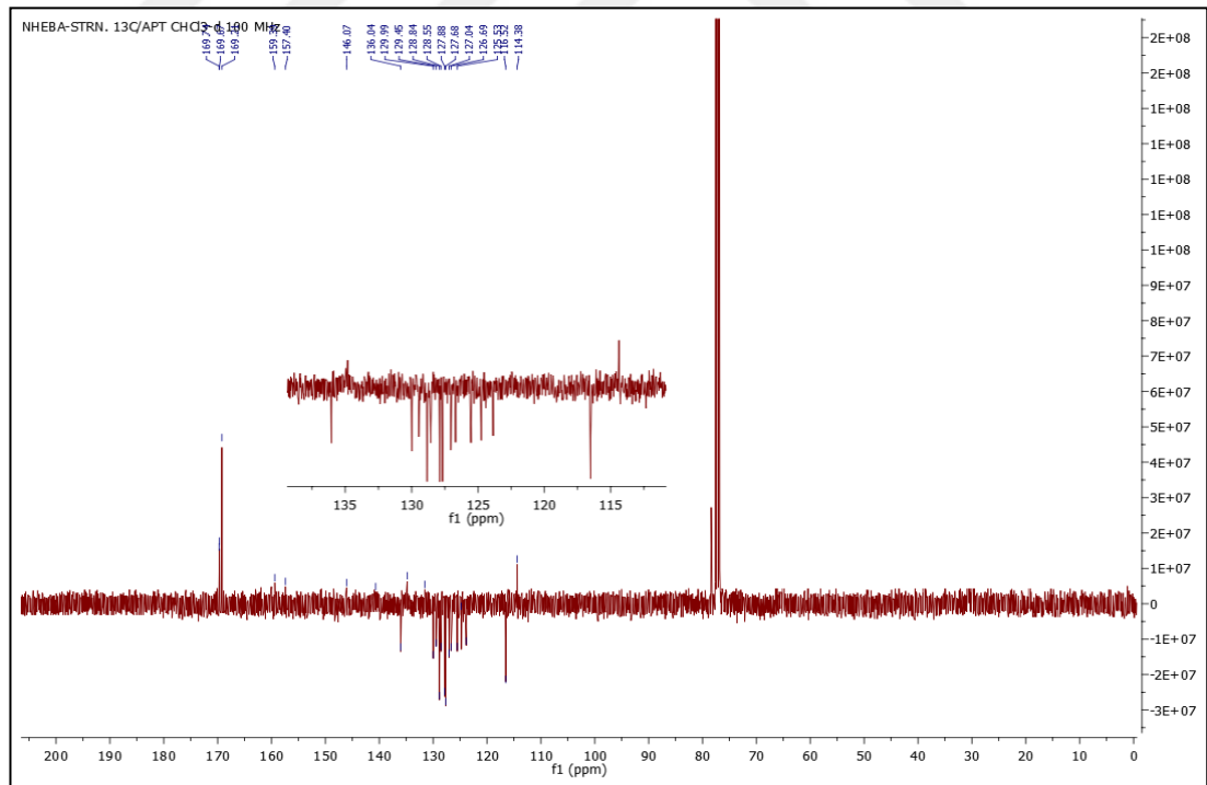
Şekil 4.47. Bileşik 4'ün 13 C NMR/APT spektrumu (CHCl 3 -d)
