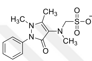
Novalgin 73
