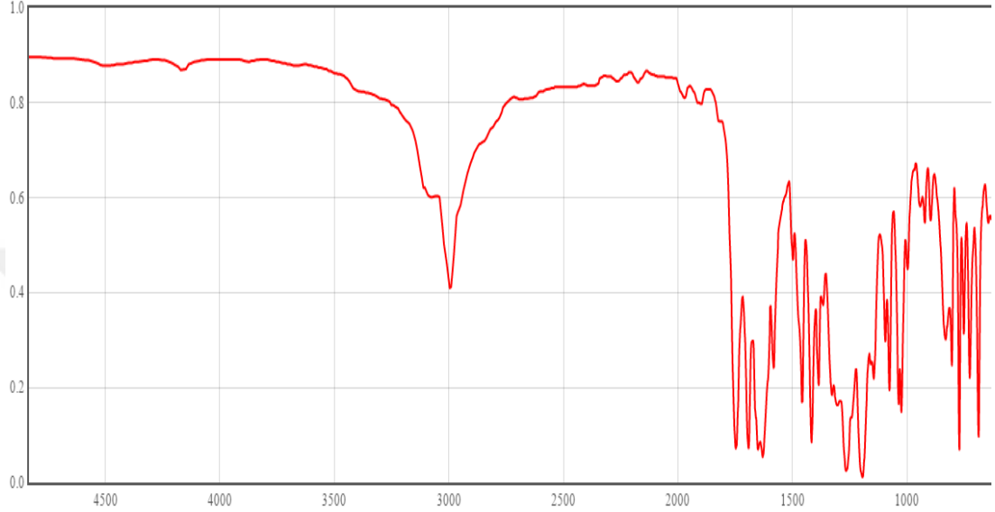
Şekil 4.4. Etil benzoilasetat bileşiğinin FTIR spektrumu
