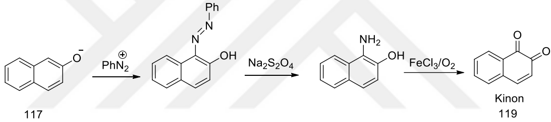
Şekil 1.57. Kinon (119) sentezi
