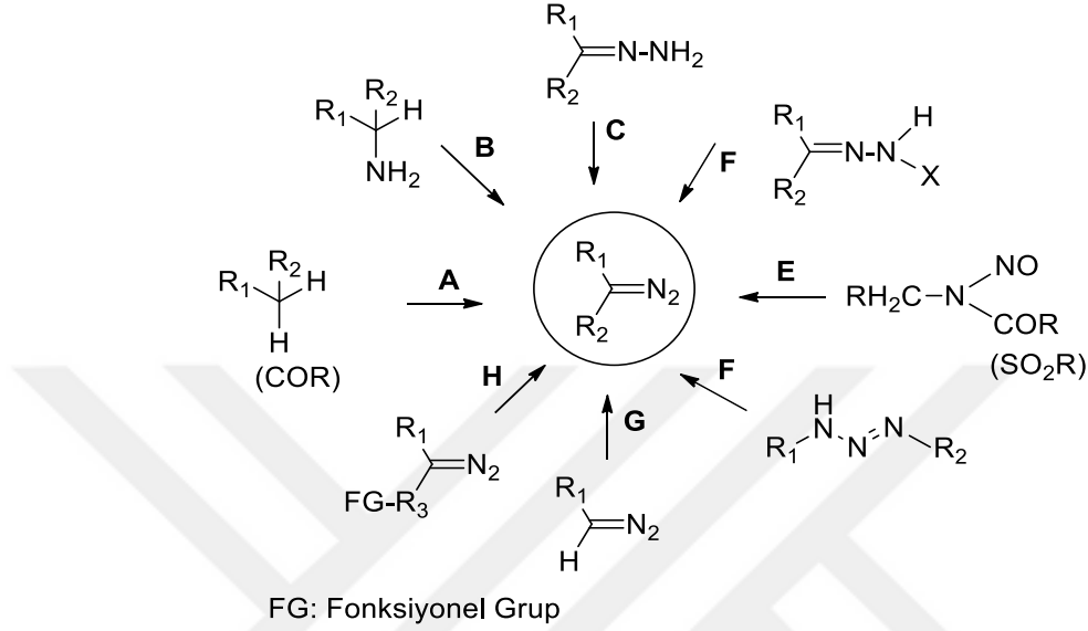
Şekil 1.58. Diazo bileşiklerinin modern sentez yöntemleri (A: Aktive metilen ya da metin grubuna diazo-grup transferi, B: \alpha -Akseptör substitüe primer alifatik aminlerin diazolanması, C: Hidrazonların dehidrojenasyonu, D: Sülfonil hidrazonların bazla muamelesi, E: N -Alkil- N -nitroso sülfon amitlerin, karboksamitlerin, üre ve üretanların bazik ayrılması, F: Triazen parçalanması, G: Diazometil bileşiklerinde elektrofilik yer değişirme, H: Diazo bileşiklerinin sıstitüent değişimi)
