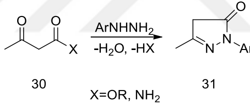
Şekil 1.10. 1-Aril-3-metil-5-pirazolonların sentezi
