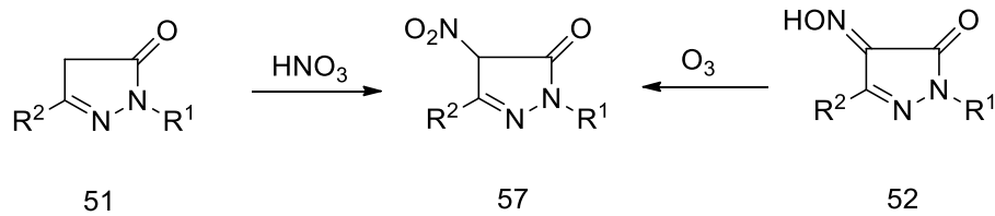
Şekil 1.26. 2-Pirazolin-5-onların nitrolanması
