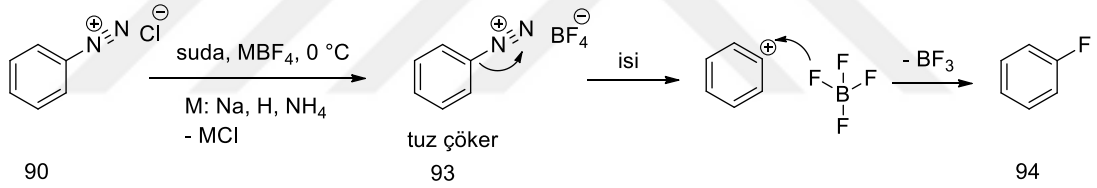
Şekil 1.44. Halojenle yer deęiřtirme
