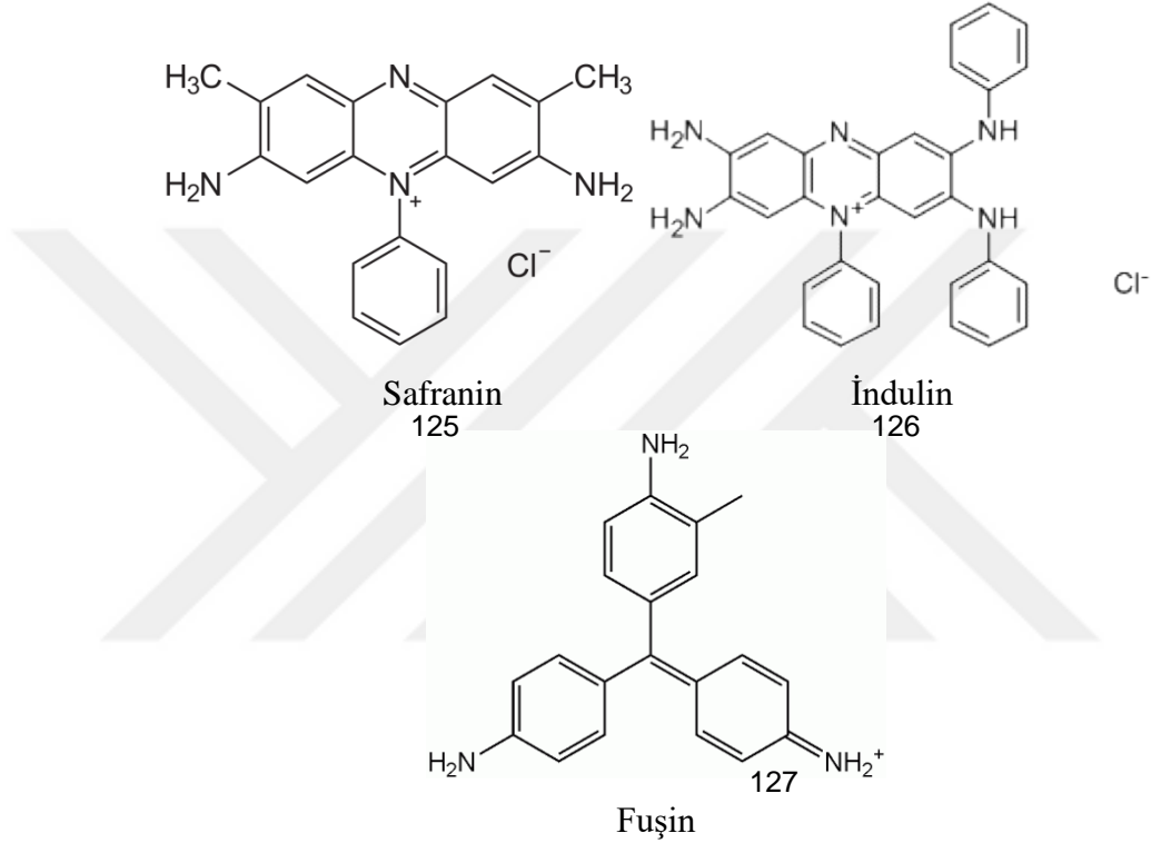
Şekil 1.61. Çeşitli sentetik boyalar
