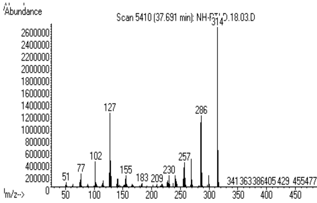
Şekil 4.40. Bileşik 3'ün GC-MS spektrumu
