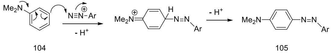
Şekil 1.49. Kenetlenme reaksiyonu
