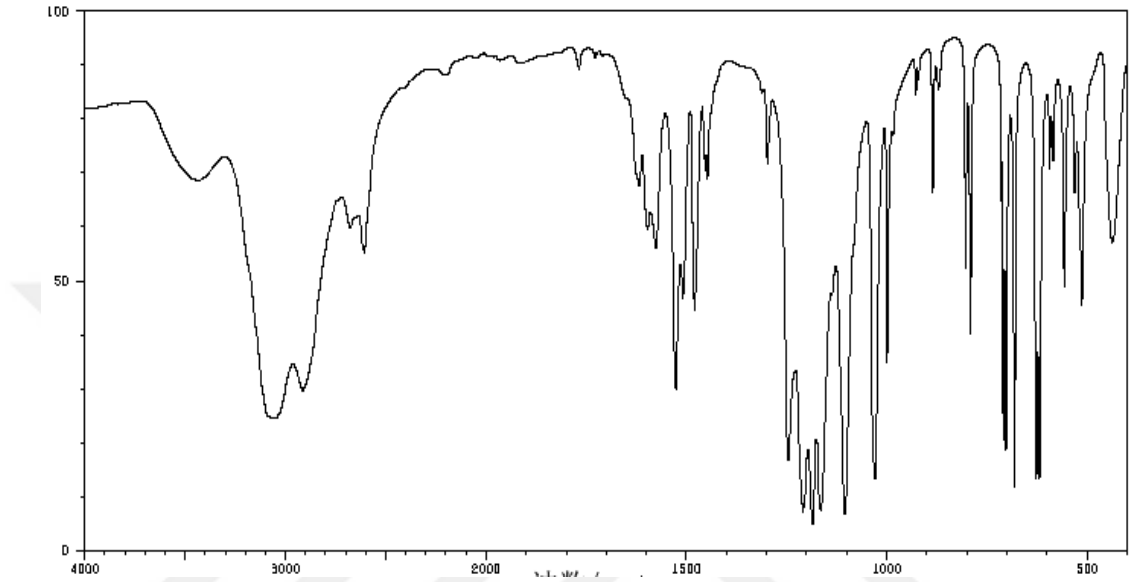
Şekil 4.15. 1-Aminobenzen-3-sülfonik asit bileşiğinin FTIR spektrumu
