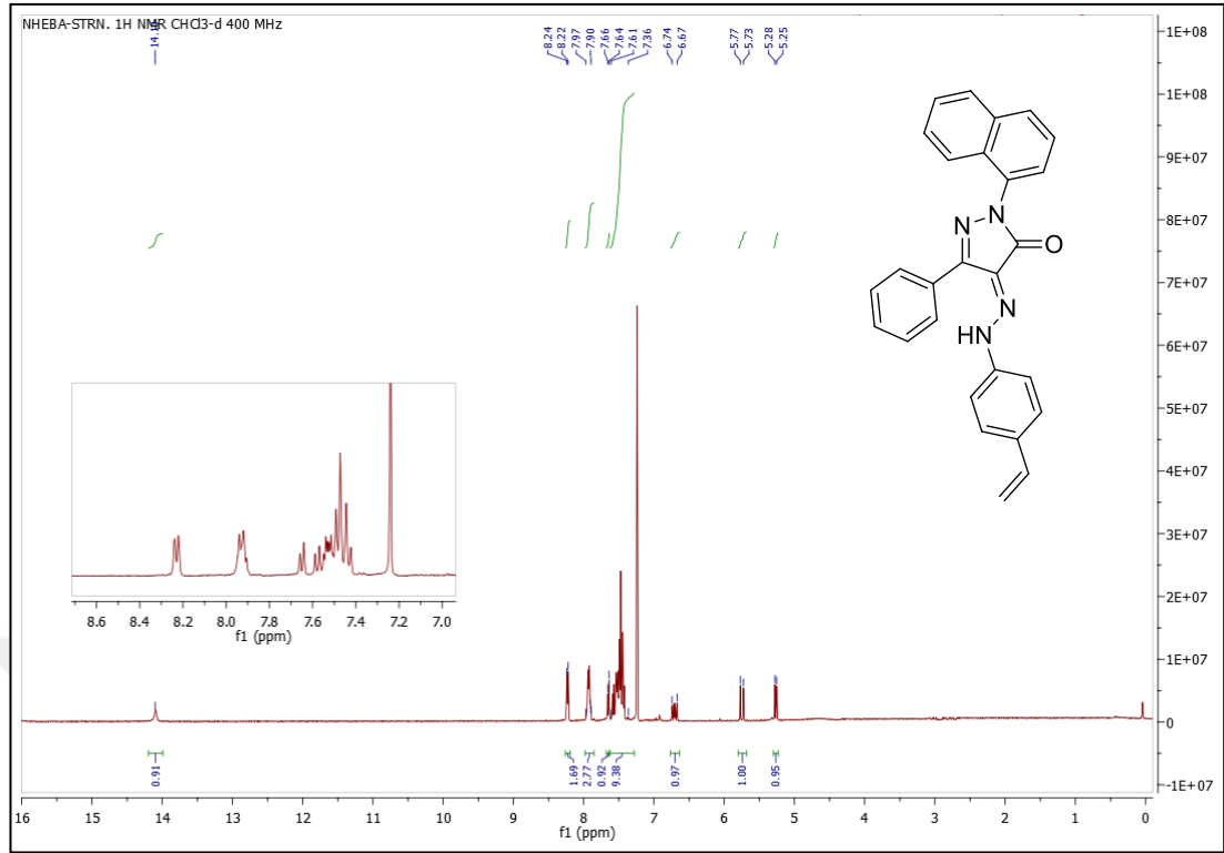
Şekil 4.46. Bileşik 4'ün 1 H NMR spektrumu (CHCl 3 -d)
