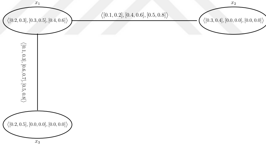
Şekil 4.37: H_1(e_1) aralık değerli neutrosophic grafı
