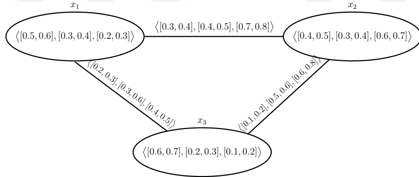
Şekil 4.1: H(e_1) aralık değerli neutrosophic grafi
