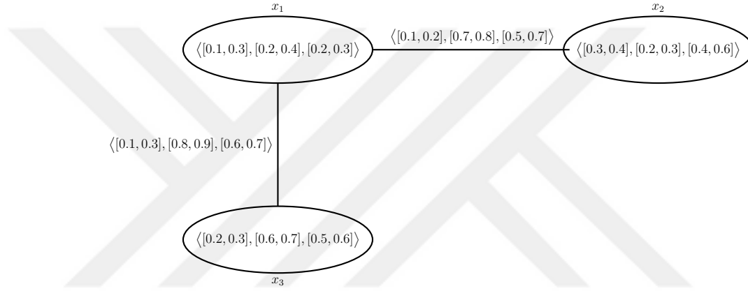
Şekil 3.13: \hat{G}_1 = (G^*, \hat{A}_1, \hat{B}_1) aralık değerli neutrosophic grafi
