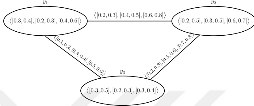
Şekil 4.11: H_2(e_2) aralık değerli neutrosophic grafi
