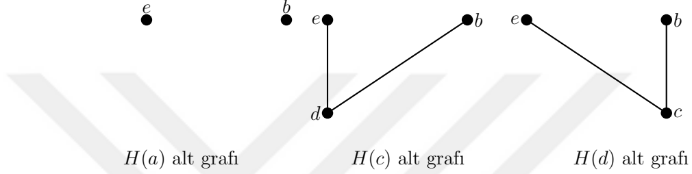
Şekil 2.2: H(a), H(c), H(d) alt grafları
