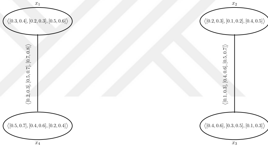
Şekil 4.16: H_1(e_2) aralık değerli neutrosophic grafi
