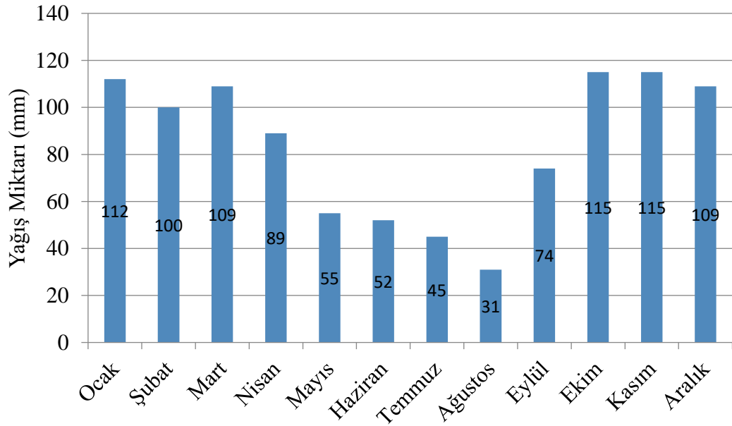
Şekil 3. 3 Fatsa İlçesi Aylık Yağış Dağılımı (Anonim, 2019c)
