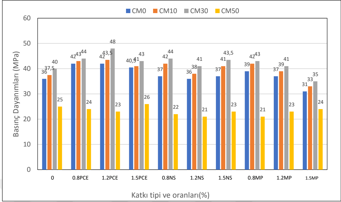
Şekil 4.7 Harçların ortalama basınç dayanımlarının değışimleri
