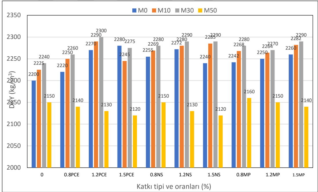
Şekil 4.8 Harçların yerdeğıştirme ve katkı oranlarına göre ortalama DKY değışimleri
