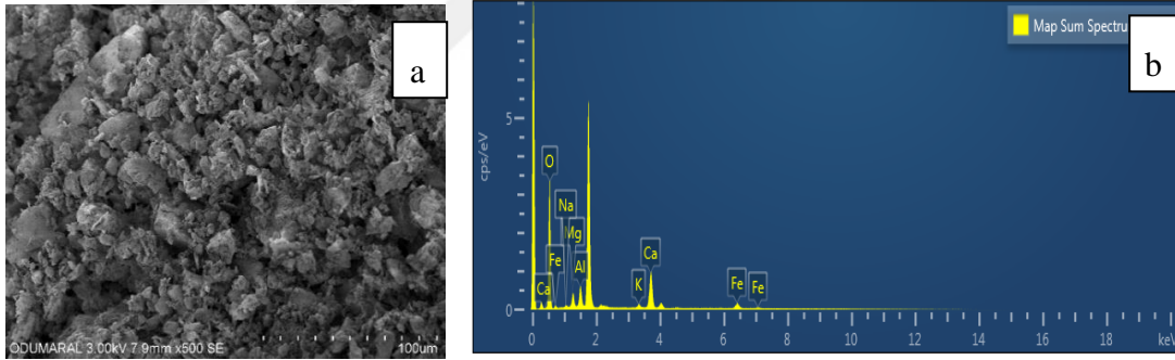
Şekil 4.5 Kalsine marnın SEM fotoğrafı (a) ve element spektrumu (b) (600°C)
