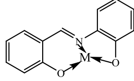
ONO tipi ligand
