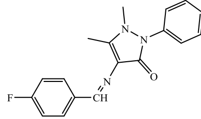
4-(4-florobenzilidinamino)-1,2-dihidro-2,3-dimetil-1-fenilpirazol-5-on
