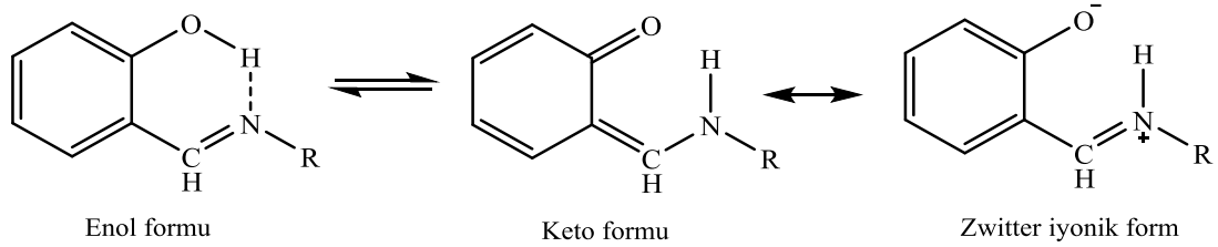
Şekil 2.6 İmin Grubuna Aromatik Halkada orto Pozisyonunda Komşu Olan Bir –OH Grubunun Keto-Enol Tautomerisi
