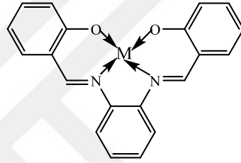
N 2 O 2 tipi ligand
