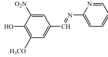
N-(pidil)-3-metoksi-4-hidroksi-5-nitrobenzaldimin
