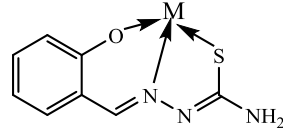
NS tipi ligand
