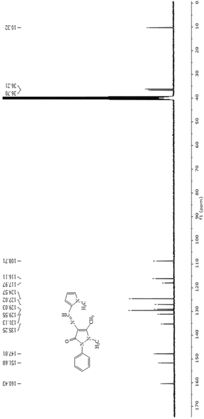
EK 3.1 Bileşik 3a için DMSO- d 6 İçerisindeki 13 C NMR Spektromu
