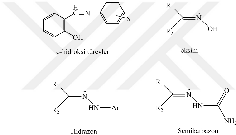
Şekil 2.2 Kararlı ve Hidrolize Dayanıklı Schiff Baz Türevlerinin Genel Yapısı
