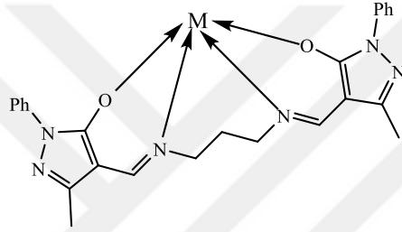
N 2 O 2 tipi ligand
