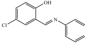
4-kloro-2-((fenilimino)metil)fenol
