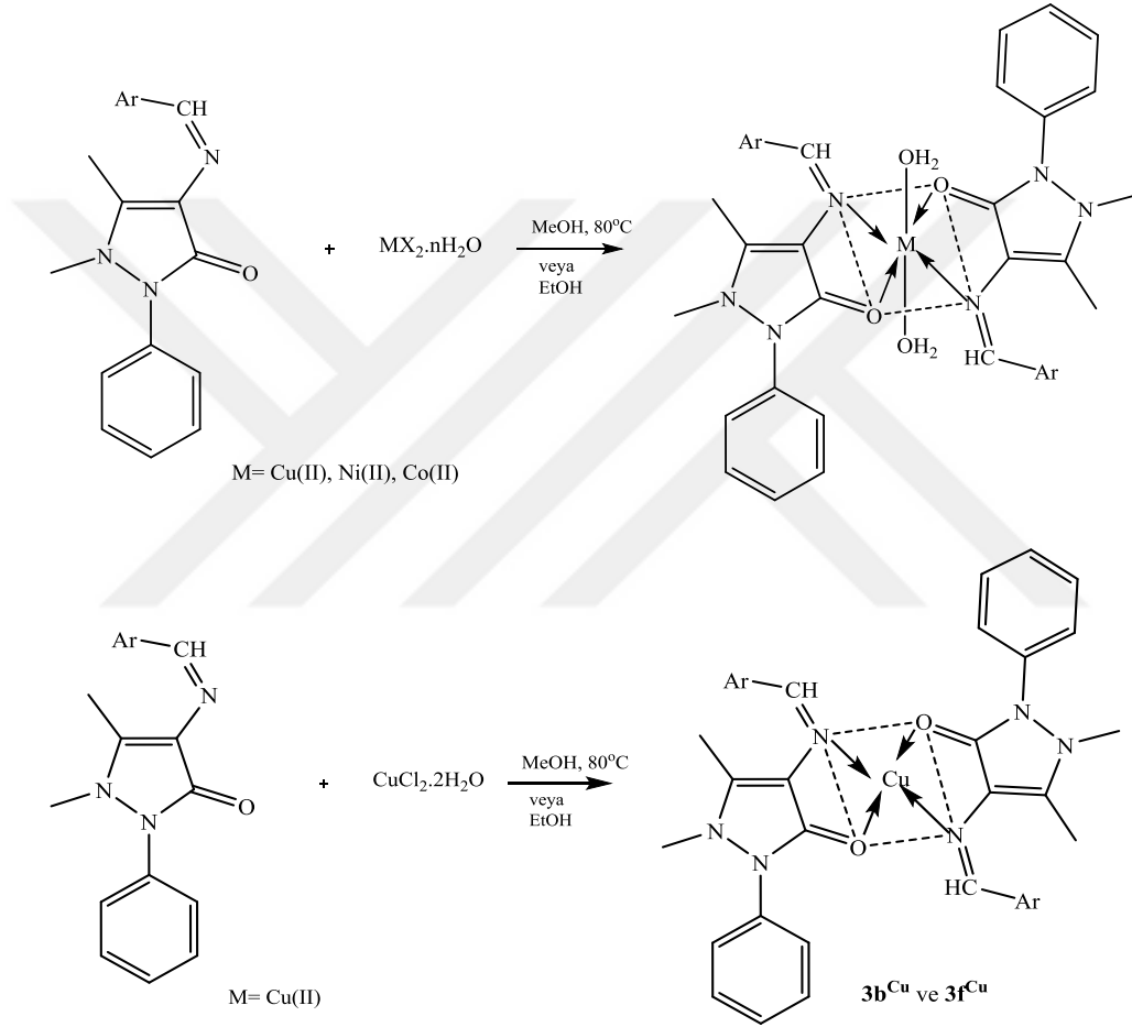
Şekil 3.2 Tez Kapsamında Elde Edilen 4-Aminoantipirin Türevli Schiff Baz Komplekslerinin Genel Sentez Şeması
