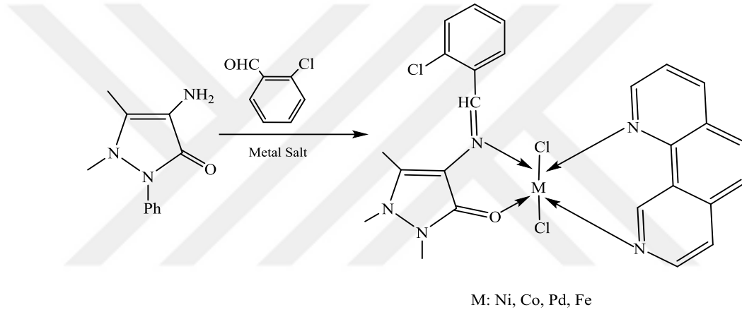
Şekil 2.16 4-Aminoantipirin Schiff Bazı Metal Komplekslerinin Oktahedral Yapısı
