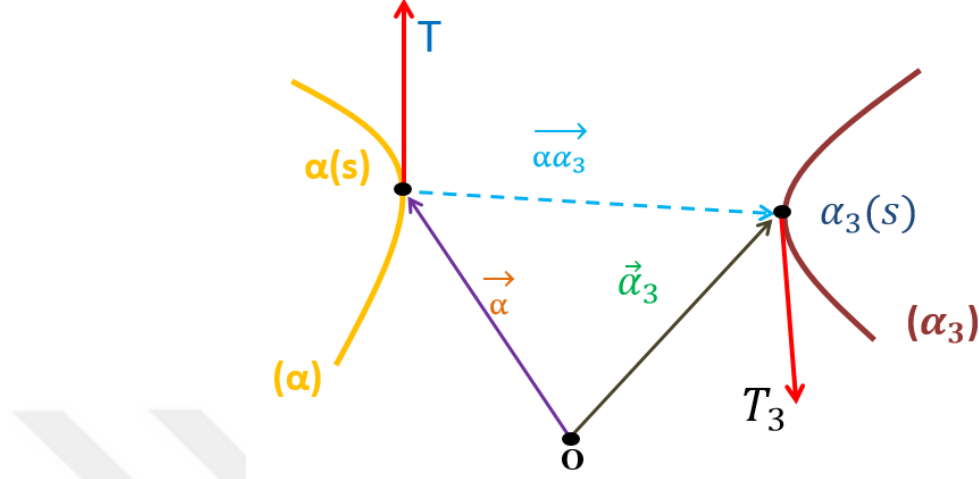
Şekil 4.7: \alpha ile \alpha_3 eğrisi sabit genişlikli eğri çifti oluşturmaz.
