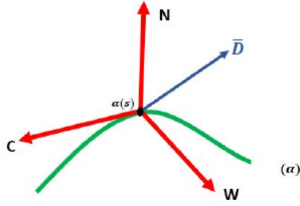
Şekil 3.2: \bar{D} alternatif Darboux vektörü
