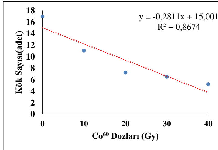
Şekil 4.9 Isabella Çeşidinde Co 60 Uygulama Dozları (Gy) ile Kök Sayısı (adet) Arasındaki Regresyon İlişki Grafiği
