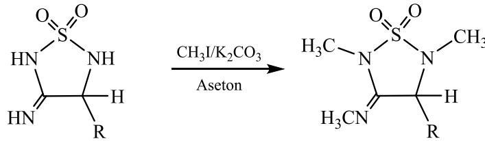
Şekil 2.19 Sülfamidlerin Metillenmesi
