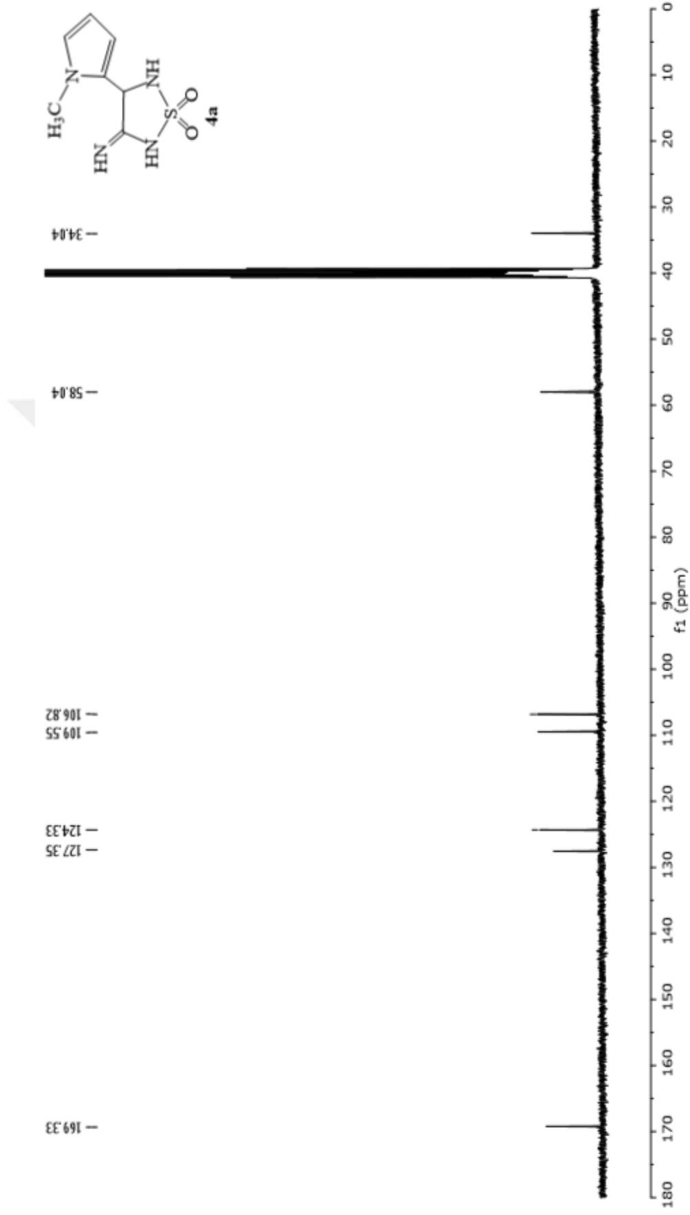
Şekil 4.3 3-İmino-4-(1-Metil-1 H -Pirrol-2-il)-1,2,5-Tiyadiazolidin 1,1-Dioksit ( 4a ) Bileşiğinin DMSO- d 6 daki 13 C NMR Spektrumu
