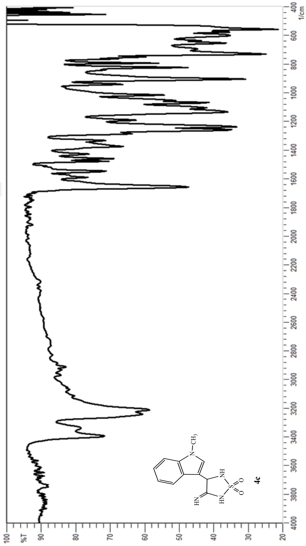
Şekil 4.7 3-İmino-4-(1-Metil- H -İndol-3-il)-1,2,5-Tiyadiazolidin 1,1-Dioksit ( 4c ) Bileşiğinin IR Spektrumu
