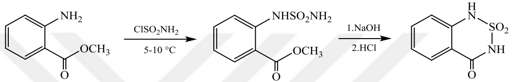
Şekil 2.5 Sülfamoil Klorür ve Sübstütüe Anilininle Açık ve Halkalı Sülfamidlerin Sentezi
