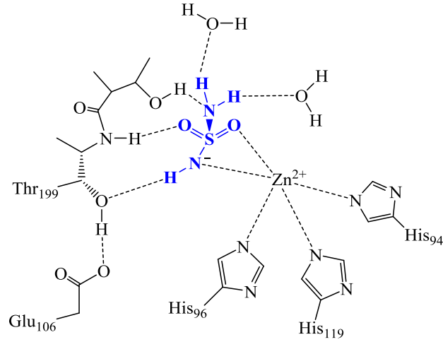
Şekil 2.33 Enzim İnhibitörü Olarak Sülfamidin Bağlanma Merkezleri
