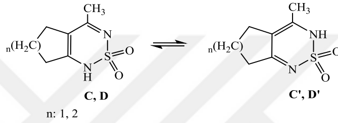
Şekil 2.18. Bazı Halkalı Sülfamidlerin Tautomerleşme Dengeleri
