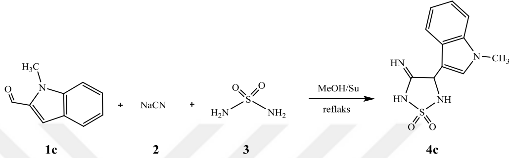
Şekil 3.4 Bileşik 4c için Sentez Reaksiyonu
