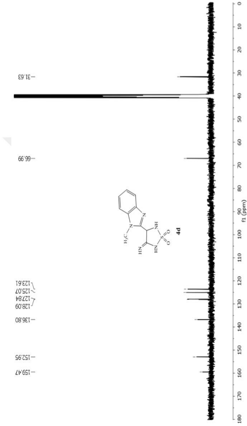
Şekil 4.12 3-İmino-4-(1-Metil-1 H -Benzo[d]imidazol-2-il)-1,2,5-Tiyadiazolidin 1,1-Dioksit ( 4d ) Bileşiğinin DMSO- d 6 daki 13 C Spektrumu
