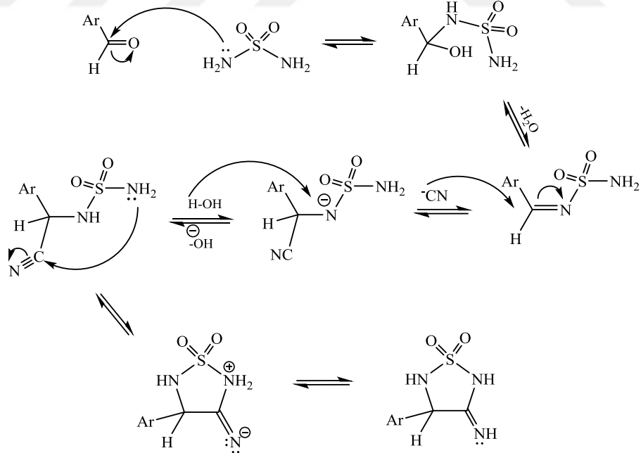
Şekil 5.1 3-İmino-4-Sübstitüe-1,2,5-Tiyadiazolidin-1,1-Dioksitlerin Eldesi için Önerilen Reaksiyon Mekanizması
