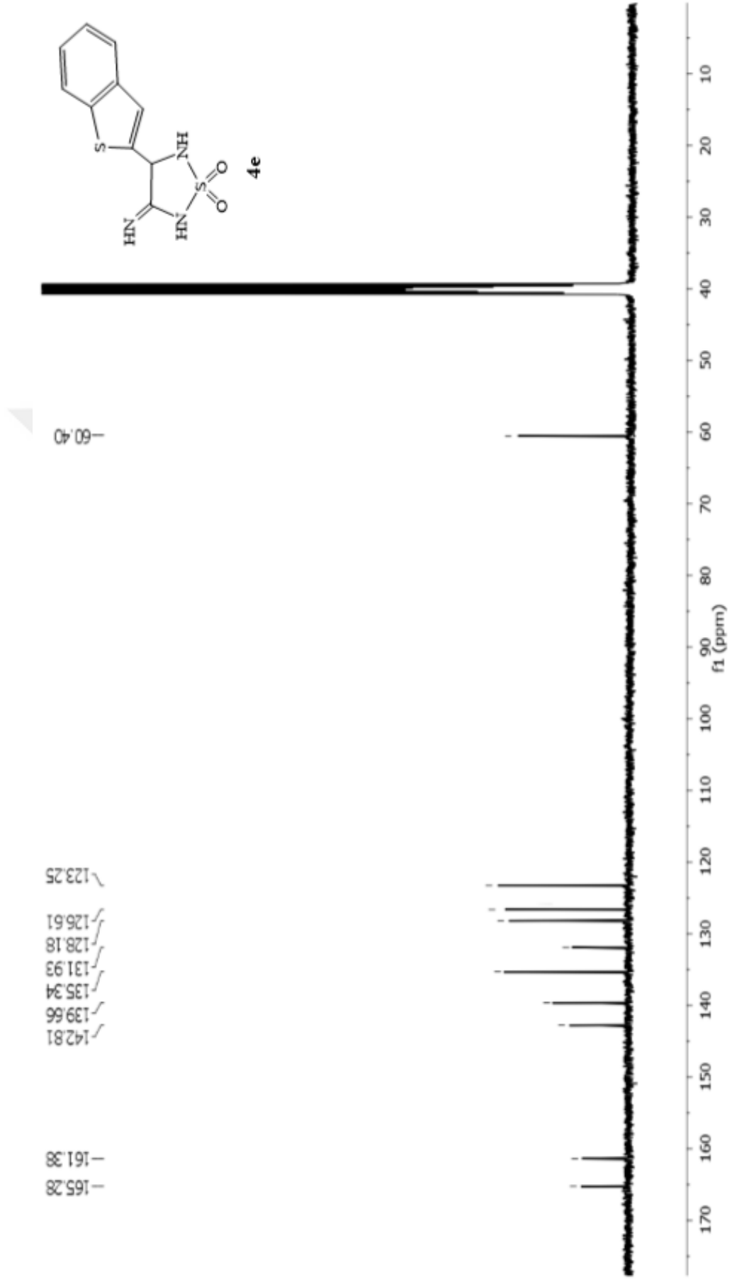
Şekil 4.15 3-İmino-4-(Benzo[ b ]tiyofen-2-il)-1,2,5-Tiyadiazolidin 1,1-Dioksit (4e) Bileşiğinin DMSO- d 6 daki 13 C NMR Spektrumu
