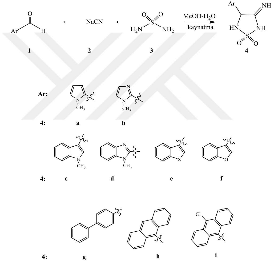
Şekil 3.1 Tez Kapsamında Sentezlenen 3-İmino-4-Süstitüe Sülfahaydantoin Bileşiklerinin Genel Sentez Şeması
