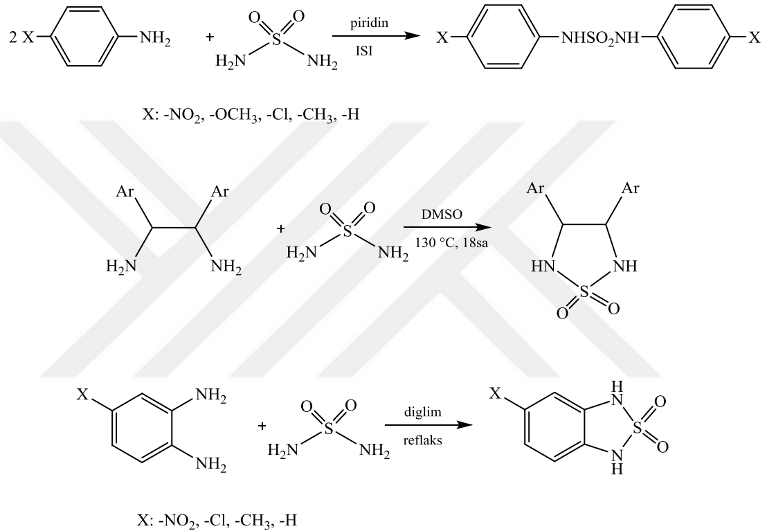
Şekil 2.8 Amin Değişimi Reaksiyonuyla Sentezlenen Bazı Sülfamidler
