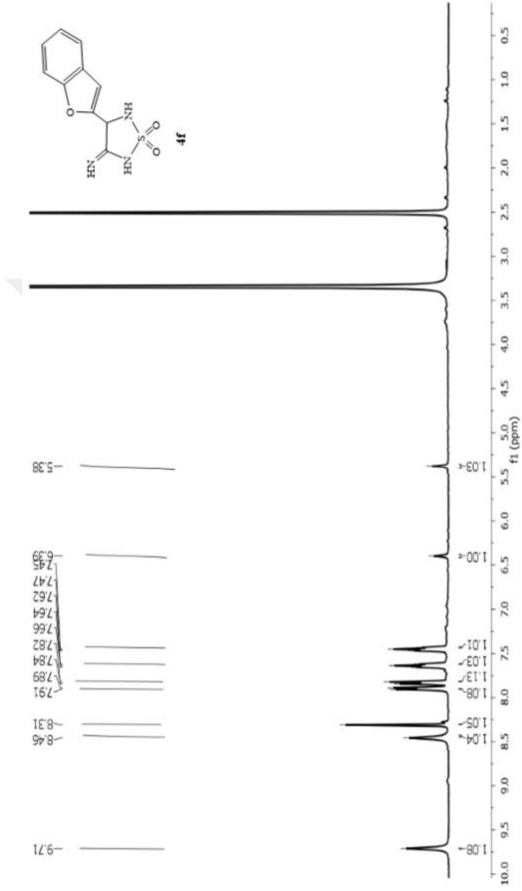
Şekil 4.17 3-İmino-3-(Benzofuran-2-il)-1,2,5-Tiyadiazolidin 1,1-Dioksit (4f) Bileşiğinin DMSO- d 6 daki 1 H NMR Spektrumu
