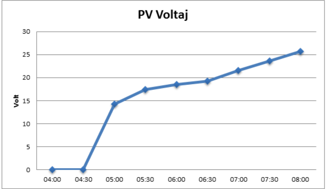
Şekil 4.5 Takip Sistemi 04:00-08:00 Panel Gerilim Değerleri
