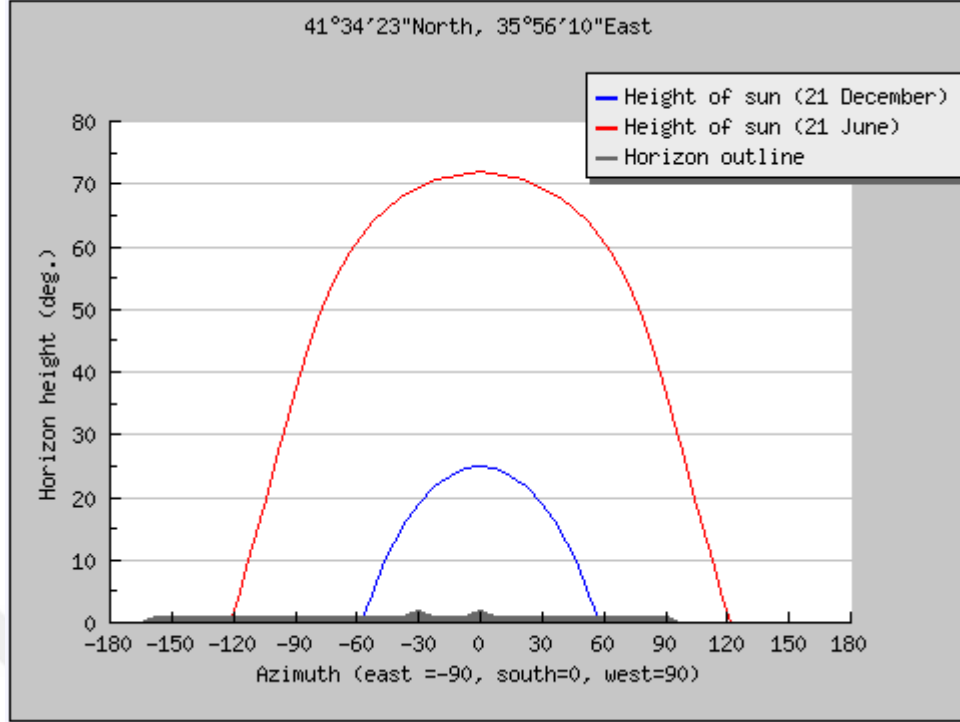
Şekil 4.15 21Aralık - 21 Haziran Güneş Yükselme Açılıları
