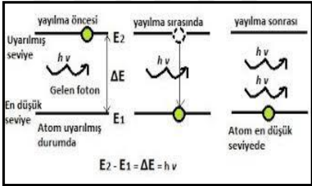
Şekil 1.1. Uyarılmış atomun bir alt enerji seviyesine foton yayarak geçişi
