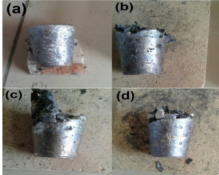
Şekil 3.3. Üretilen döküm numuneleri; (a) Al-20Si-9Fe-1.2Nb alaşımı, (b) Al-20Si-9Fe-1.2Nb-6Ni alaşımı, (c) Al-20Si-9Fe-1.2B alaşımı, (d) Al-20Si-9Fe-1.2B-6Ni alaşımı.
