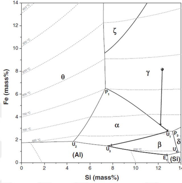
Şekil 2.5. Al-12.4Si-8Fe (kütle %) alaşımının öngörülen denge katılaşıma yolları.
