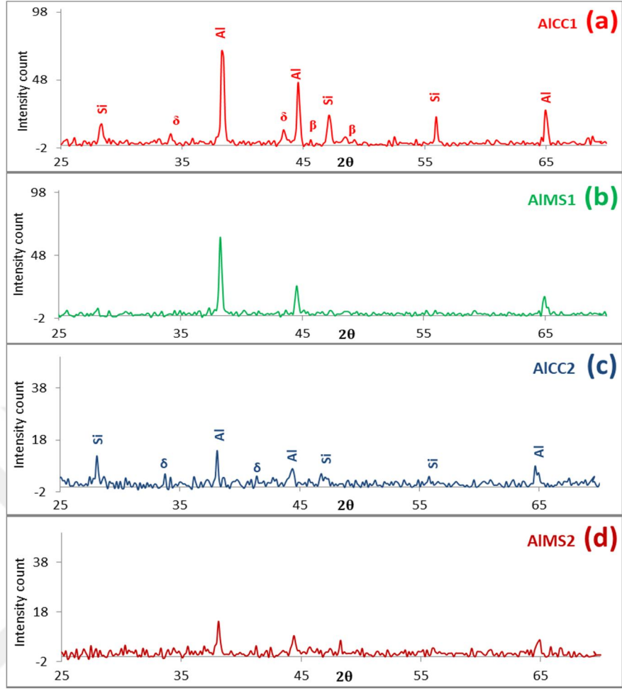
Şekil 4.22. (a) AICC1, (b) AIMS1, (c) AICC2 ve (d) AIMS2'den alınan XRD kırınım desenleri.
