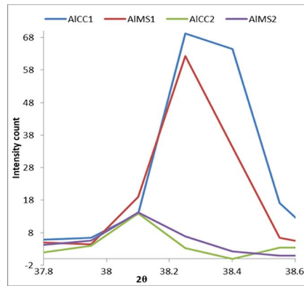
Şekil 4.23. (111) Al'in en yüksek tepe yoğunluğu kaymalarını gösteren AICC1, AICC1, AICC2 ve AICC2 örneklerinin XRD difraksiyon modelleri.
