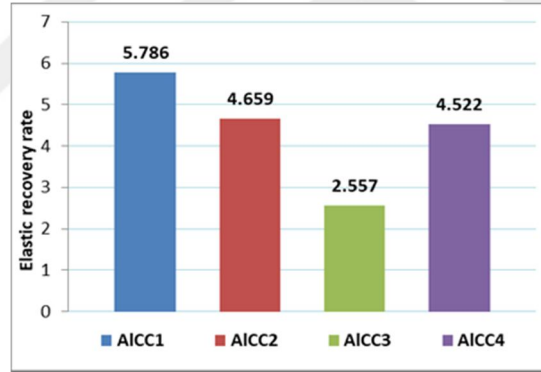
Şekil 4.21. AICC1, AICC2, AICC3 ve AICC4 alaşımlarının sünme değerindeki değişiklikler.
