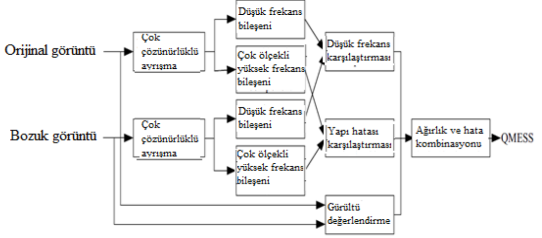
Şekil 3.7. QMESS ölçüm sisteminin şeması
