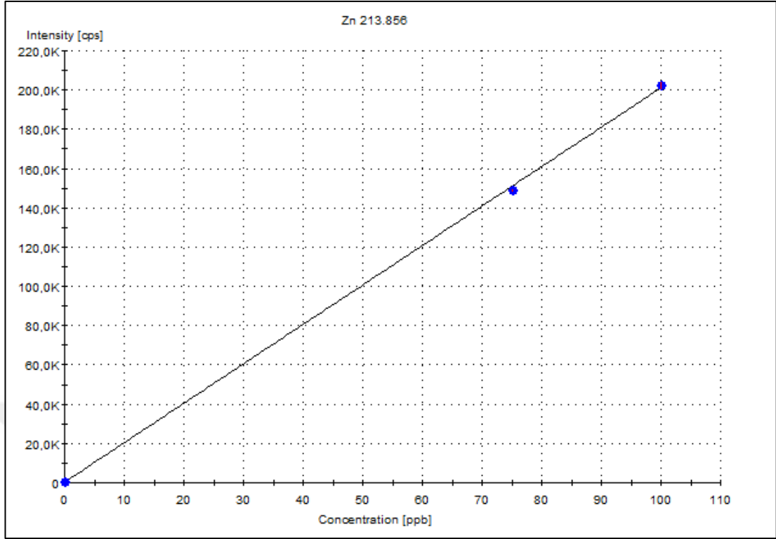
Grafik 2.6. Zn için kalibrasyon grafiđi
