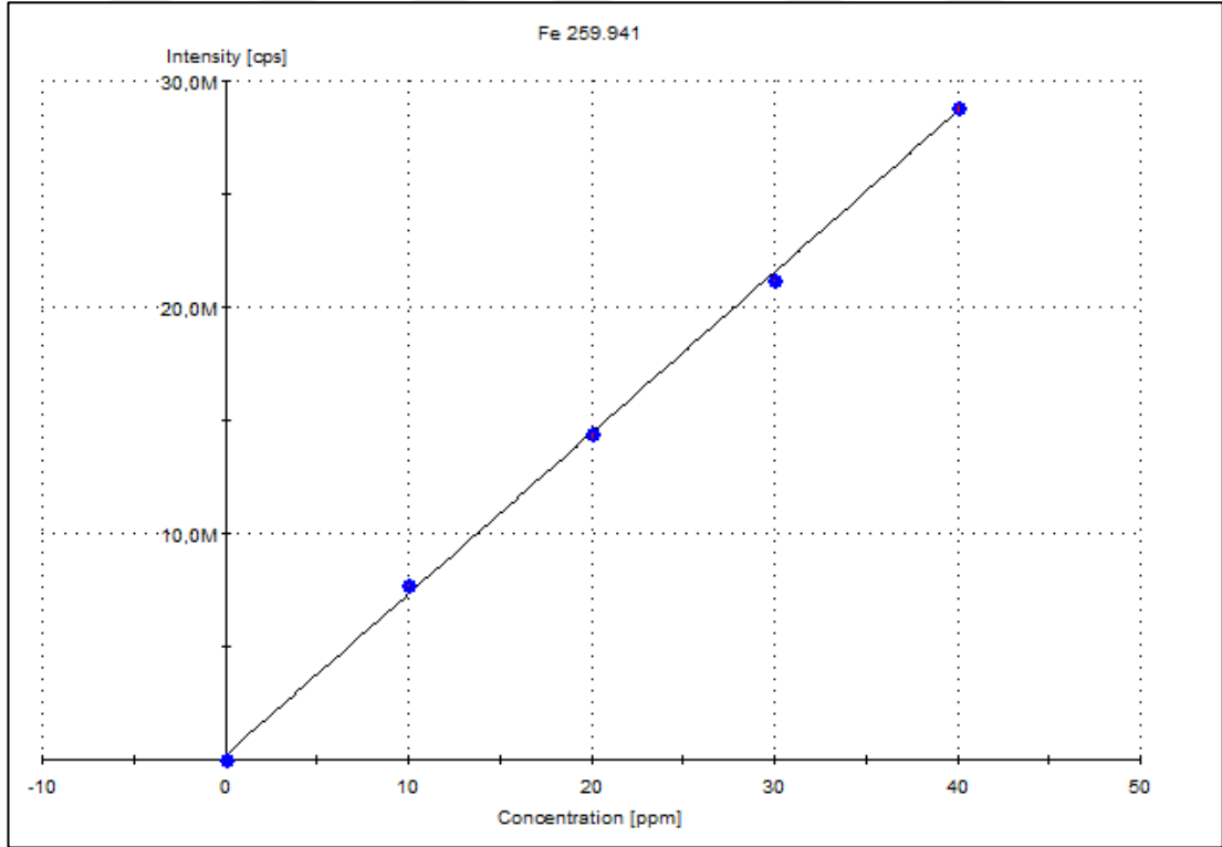
Grafik 2.7. Fe için kalibrasyon grafiđi
