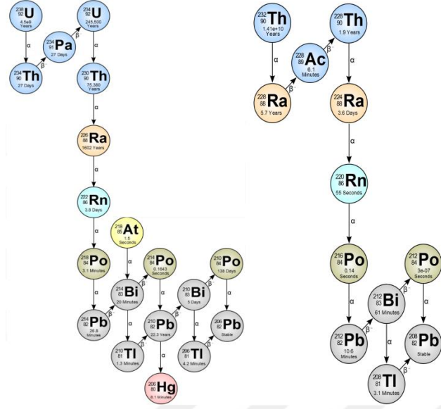
Şekil 1.2. Uranyum ve toryum serileri (URL-6)
